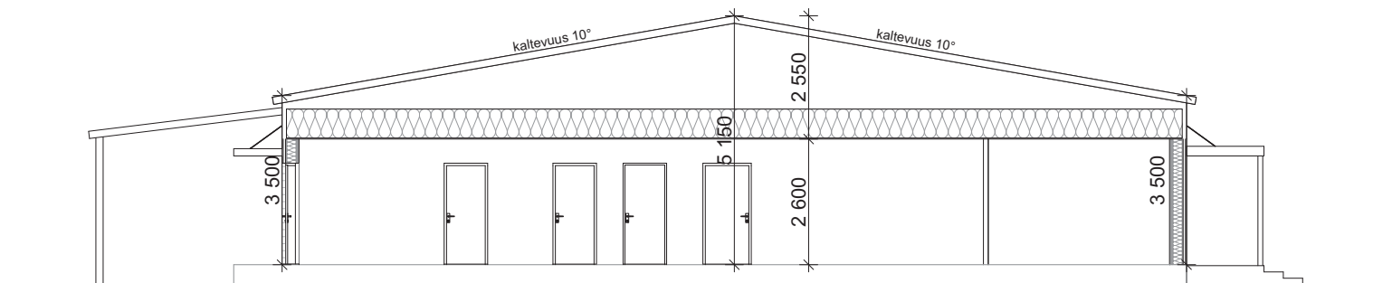
LEIKKAUS A-A
